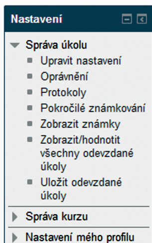
Obrázek 74 Hodnocení úloh
