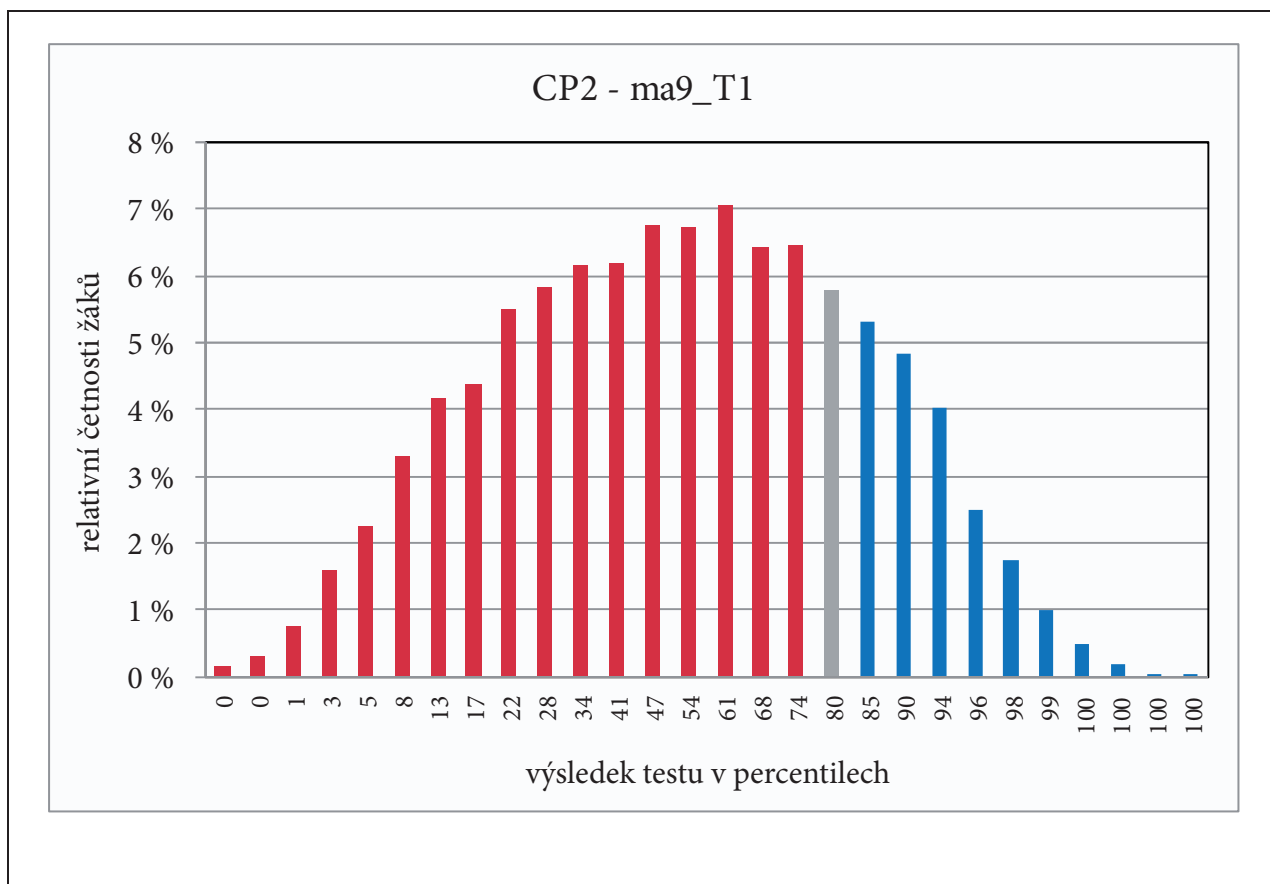
Příklad 4.68 NIQES 2013, histogramy výsledků v testu z matematiky, 9. ročník, vodorovná osa v hodnotách percentilu
