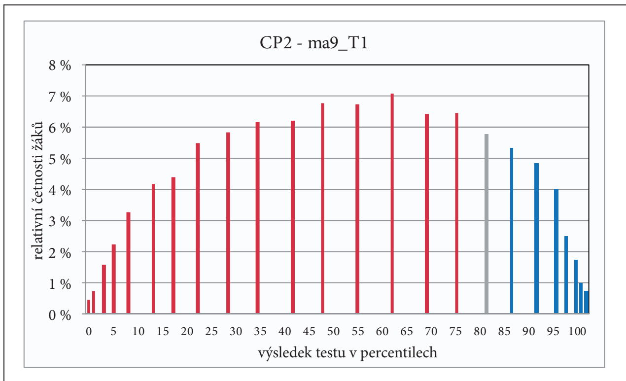
Příklad 4.68 NIQES 2013, histogramy výsledků v testu z matematiky, 9. ročník, vodorovná osa v hodnotách percentilu
